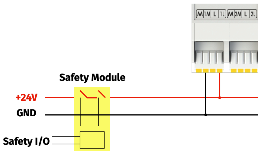
Figura 6: Doppio canale singola protezione
