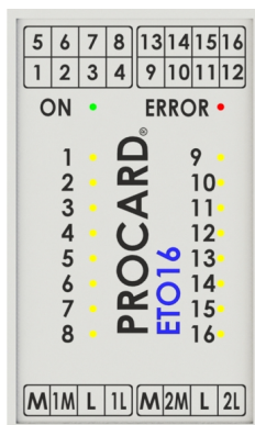
Figura 9: Led di stato
