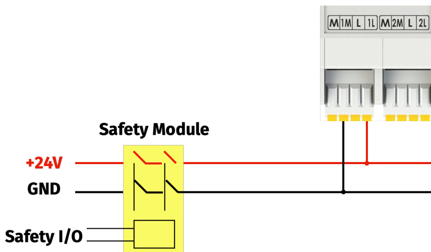
Figura 7: Doppio canale doppia protezione
