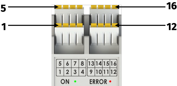
Figura 8: I/O del modulo
