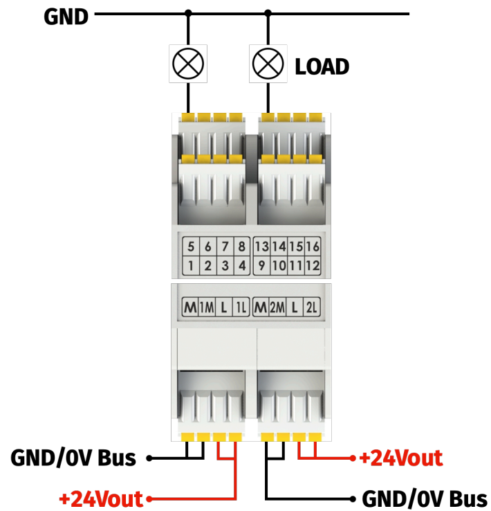
Figura 5: Alimentazione tramite bus interno
