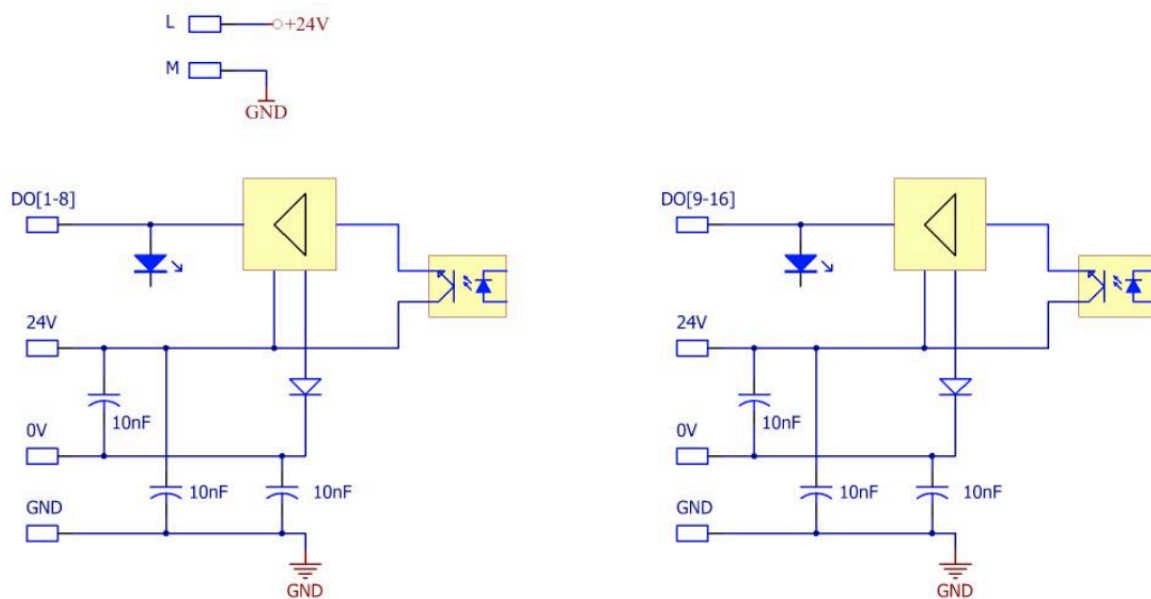
Figura 4: Diagramma schematico delle uscite
