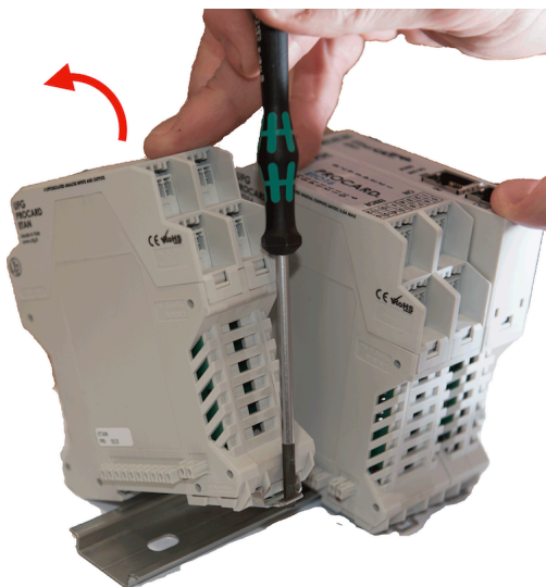
Figura 14: Rimozione del modulo da guida DIN (parte 2)
