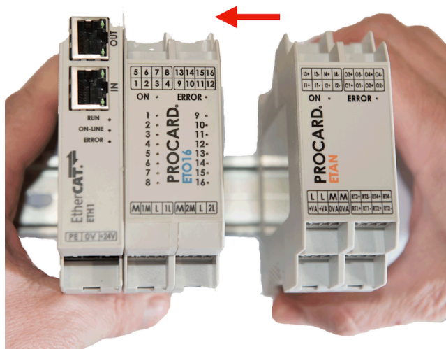
Figura 12: Collegamento elettrico dei moduli su guida DIN
