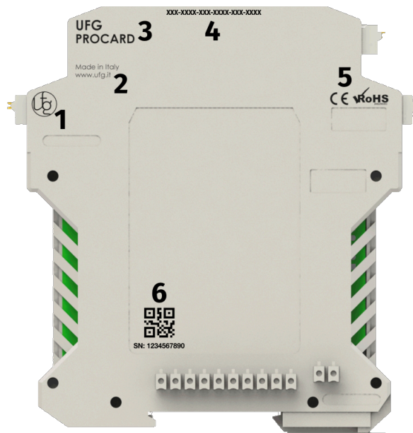
Figura 15: Simbologia del modulo
