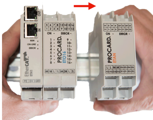
Figura 13: Rimozione del modulo da guida DIN (parte 1)
