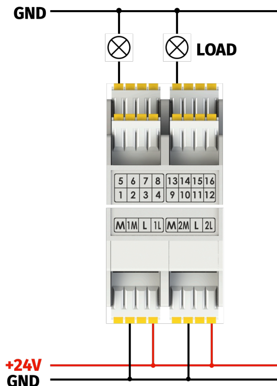
Figura 3: Alimentazione esterna
