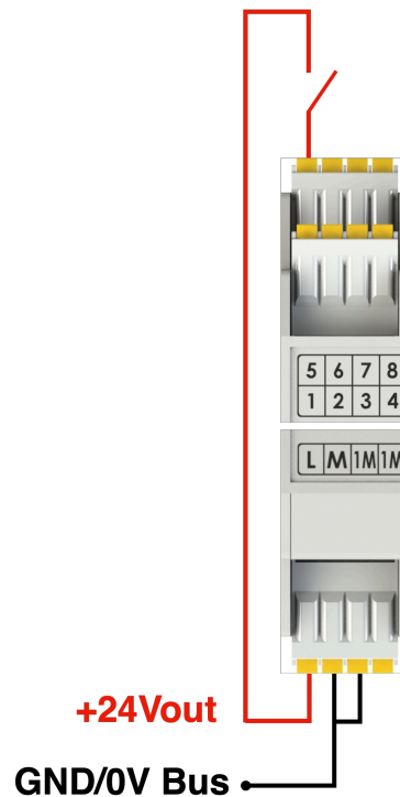
Figura 5: Alimentazione tramite bus interno
