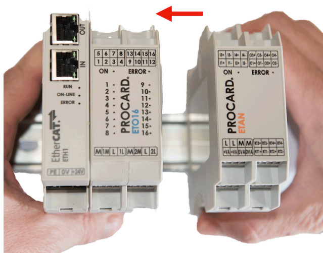
Figura 10: Collegamento elettrico dei moduli su guida DIN
