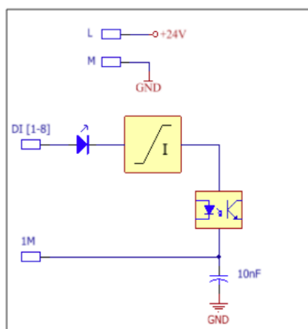
Figura 4: Diagramma schematico degli ingressi
