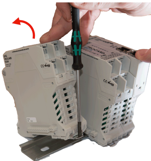
Figura 12: Rimozione del modulo da guida DIN (parte 2)
