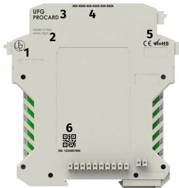
Figura 13: Simbologia del modulo
