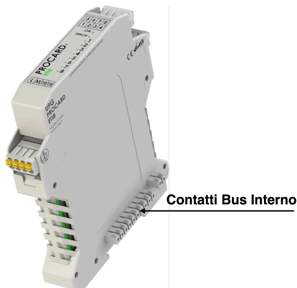
Figura 2: Connettore bus interno
