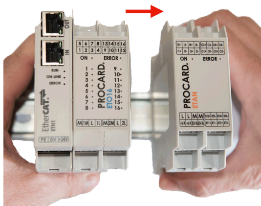
Figura 11: Rimozione del modulo da guida DIN (parte 1)
